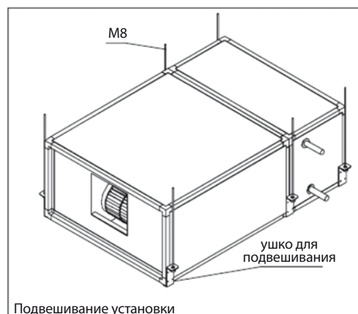
Подвешивание установки
