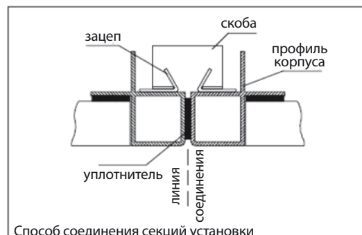
Способ соединения секций установки
