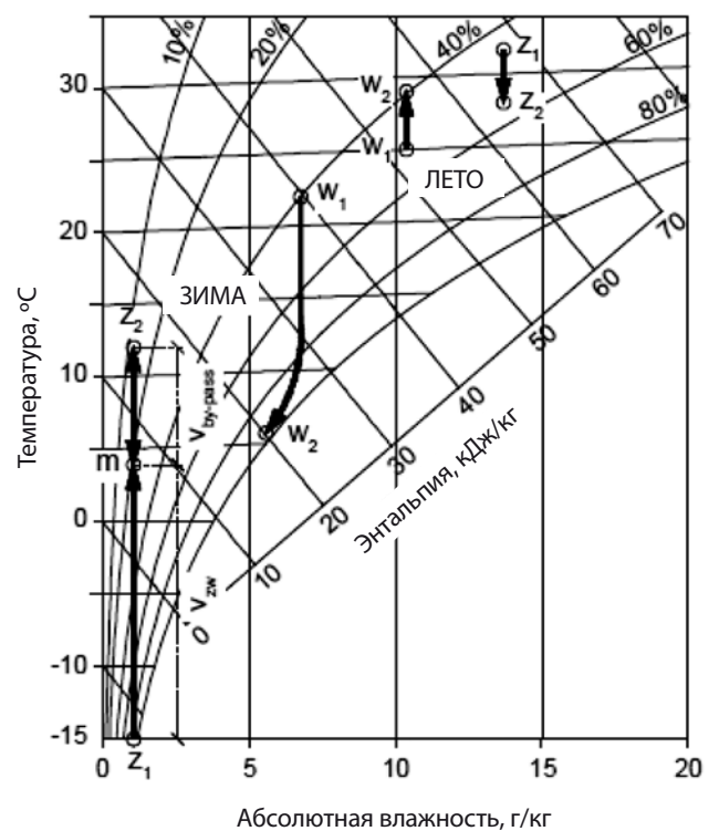
Ход процесса на графике h-x, с обледенением
