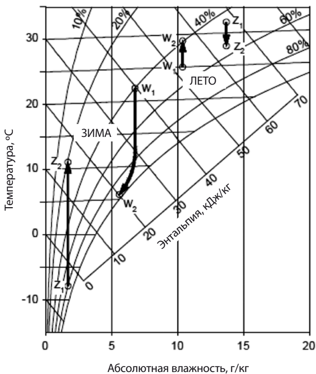
Ход процесса на графике h-x, без обледенения
