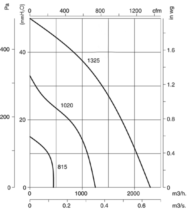
4T=1500 об/мин.
