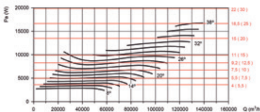
Потребляемая мощность
