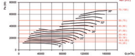
Потребляемая мощность
