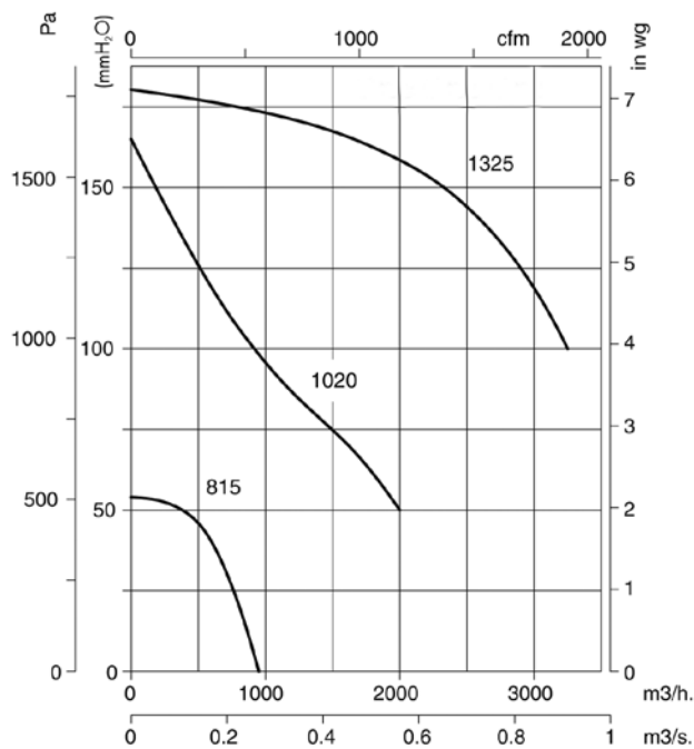
2T=3000 об/мин.
