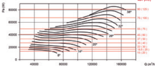
Потребляемая мощность
